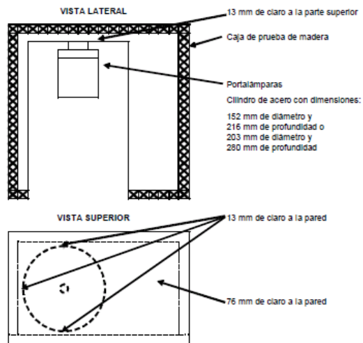
Figura 1.- Luminario de prueba
