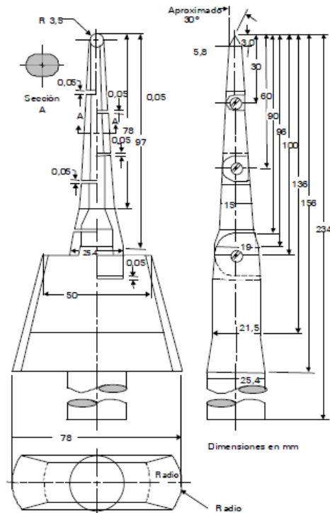
Figura 2.- Sonda de prueba articulada
